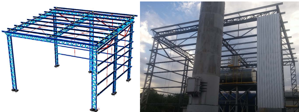
Figura 5: Perspectiva da estrutura projetada e executada – Galpão da Caldeira
