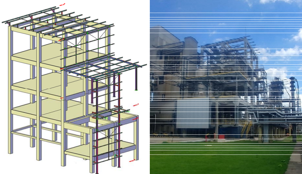
Figura 25: Perspectiva do Modelo BIM e execução da cobertura e fechamento lateral do Prédio de Purificação de HPMC
