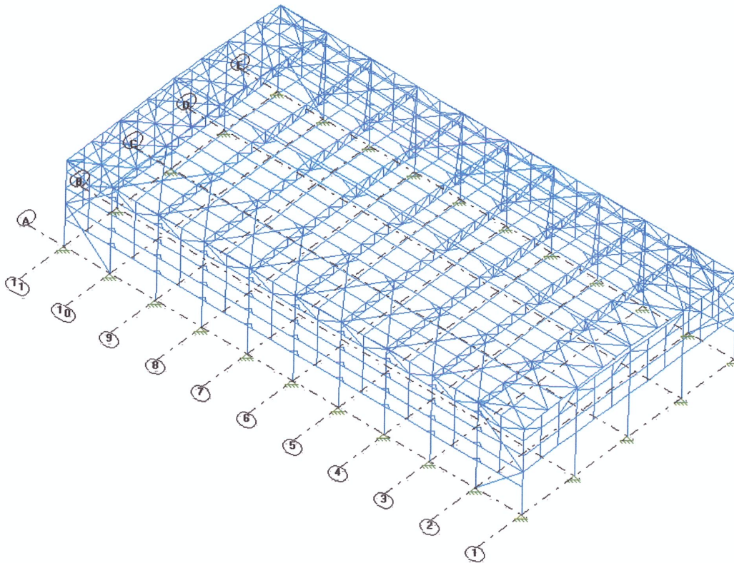
Figura 2.2: Lançamento estrutural em software de elementos finitos (Perspectiva)
