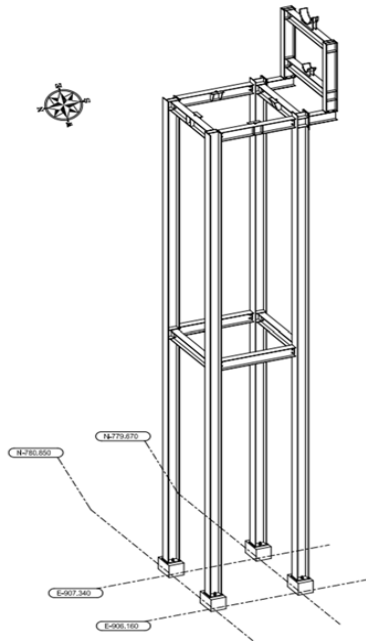
Figura 7: Perspectiva da estrutura projetada e executada – Trocador de Calor
