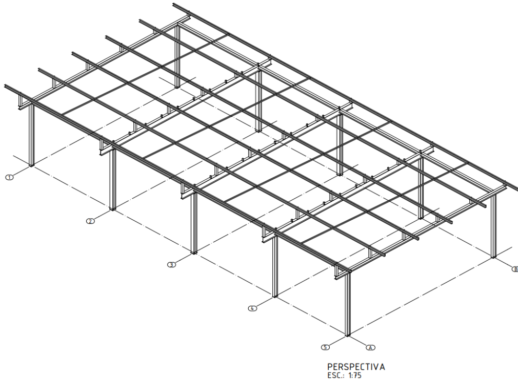
Figura 1: Elaboração dos projetos estruturais, perspectiva da estrutura metálica da casa de bombas para 12 motores
