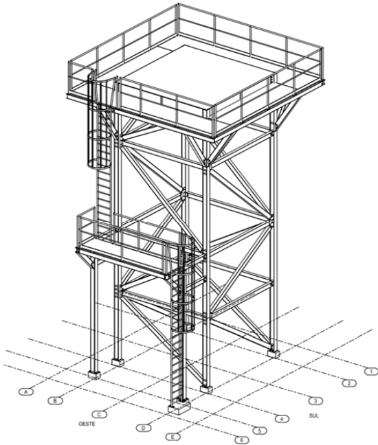
Figura 6: Perspectiva da estrutura projetada e executada – Torre Head Tank
