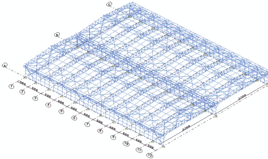
Figura 1: Perspectiva do modelo de cálculo completo (fase 3)
