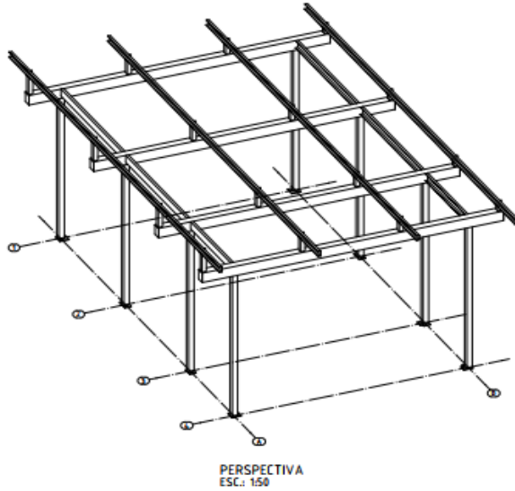
Figura 2: Elaboração dos projetos estruturais, perspectiva da estrutura metálica da casa de bombas para 2 motores
