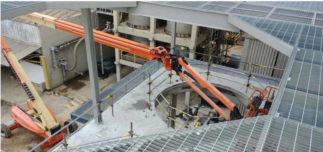
Figura 19: Montagem estrutura filtro de mangas EL114,100 e plataforma EL109,062
