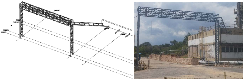
Figura 4: Perspectiva da estrutura projetada e executada – Pipe Rack
